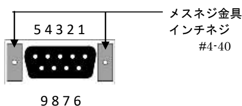
D-Sub9Pin メス型
