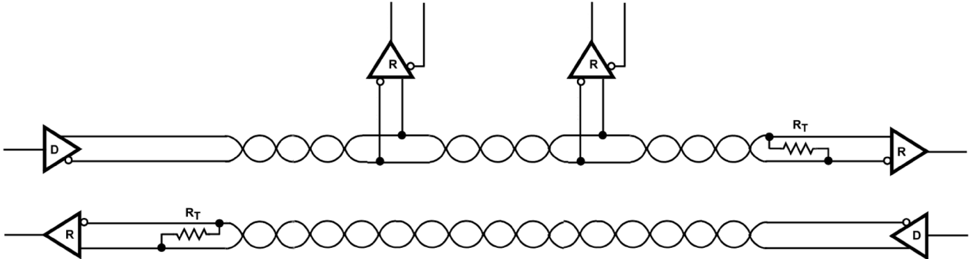
RS-485の全二重の送信・受信
