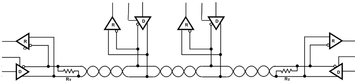
RS-485の半二重の送信・受信
